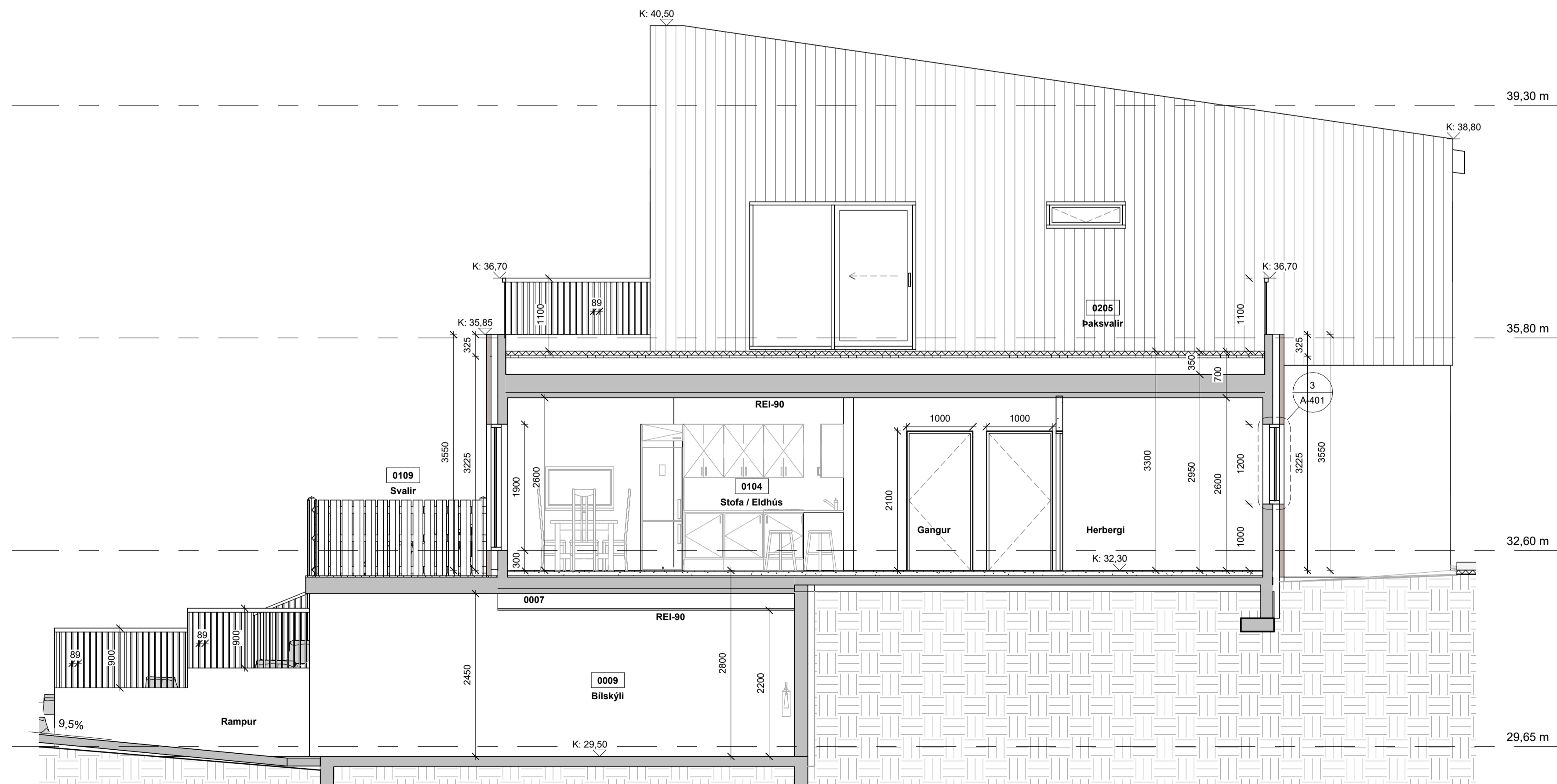
- SNIÐ F 1 : 50
