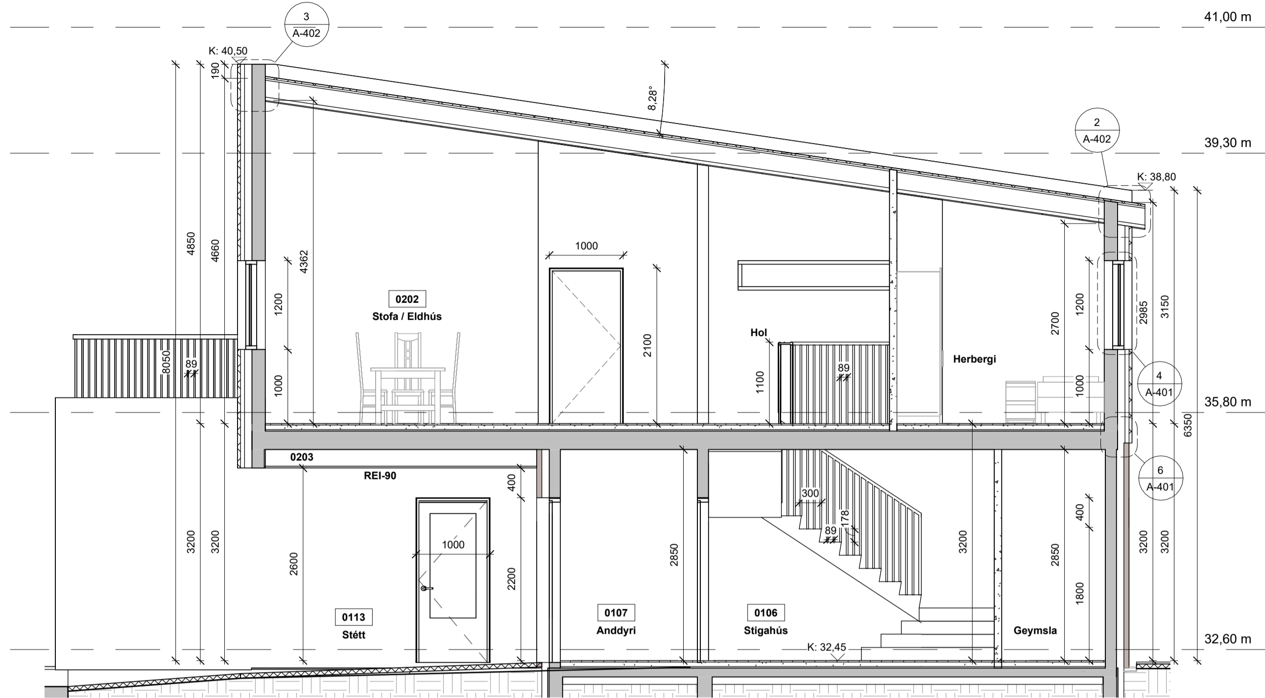
- SNIÐ D 1 : 50
