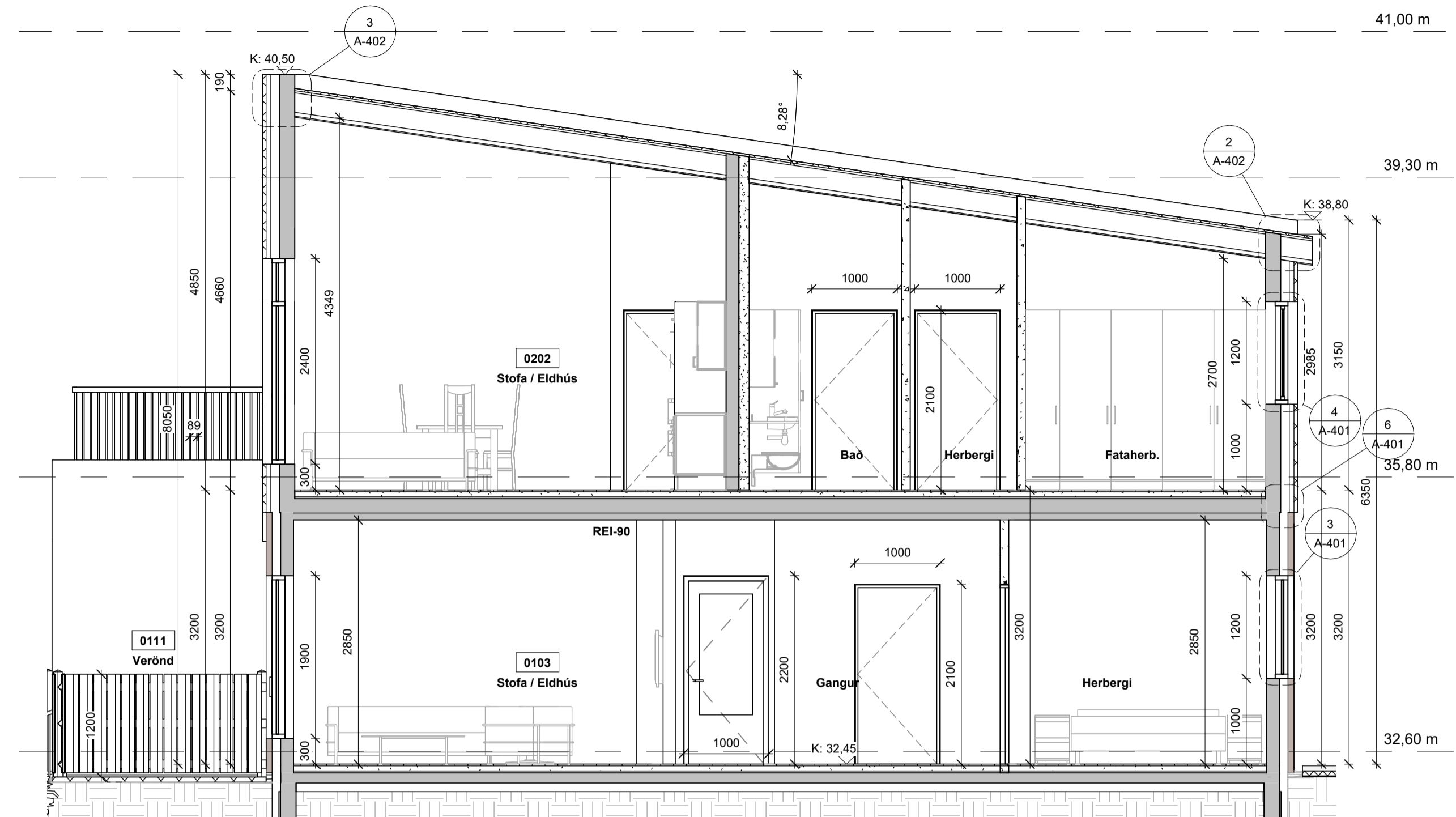
- SNIÐ E 1 : 50
