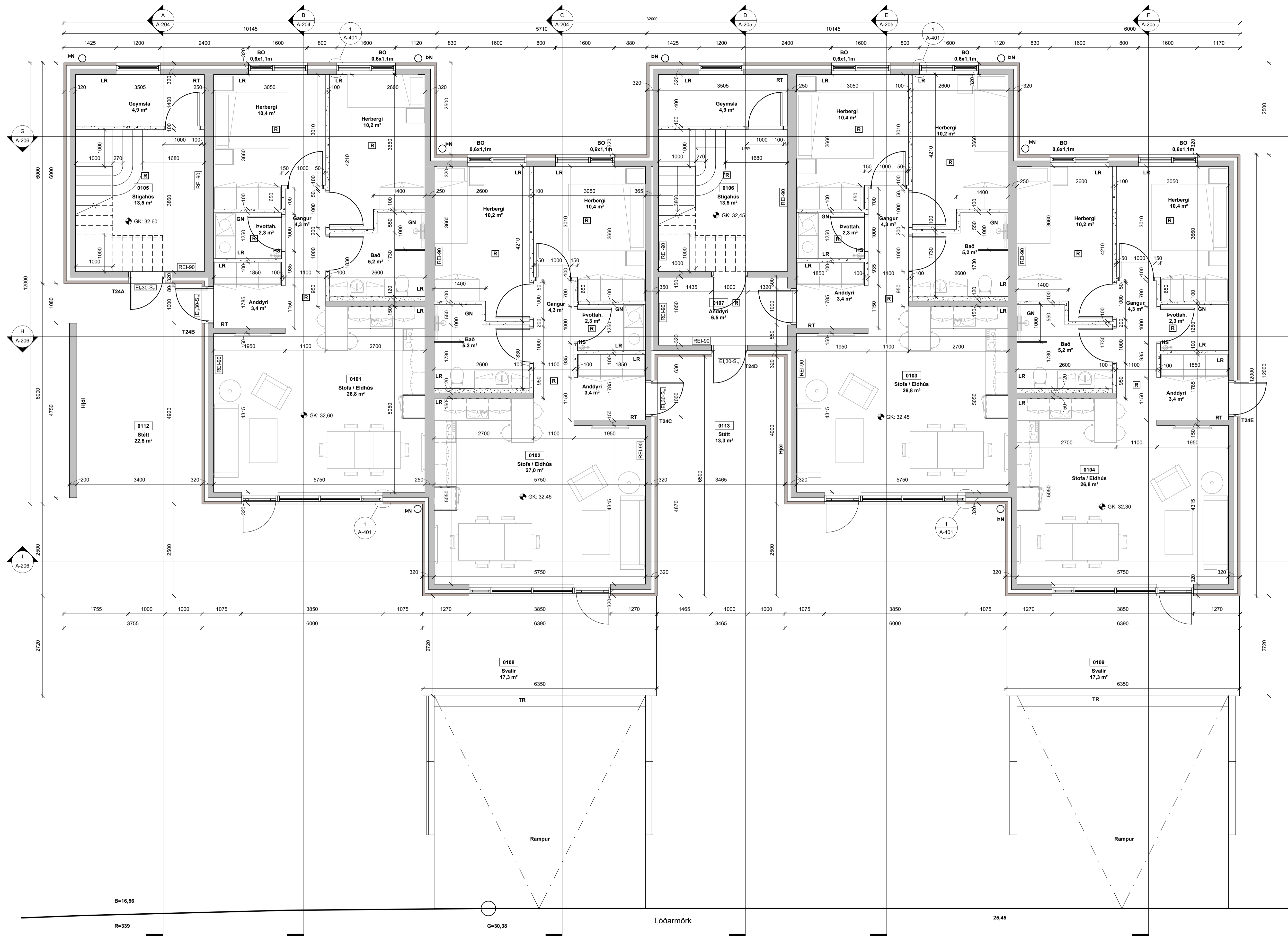
- GRUNNMYND 1. HÆÐ 1 : 50
