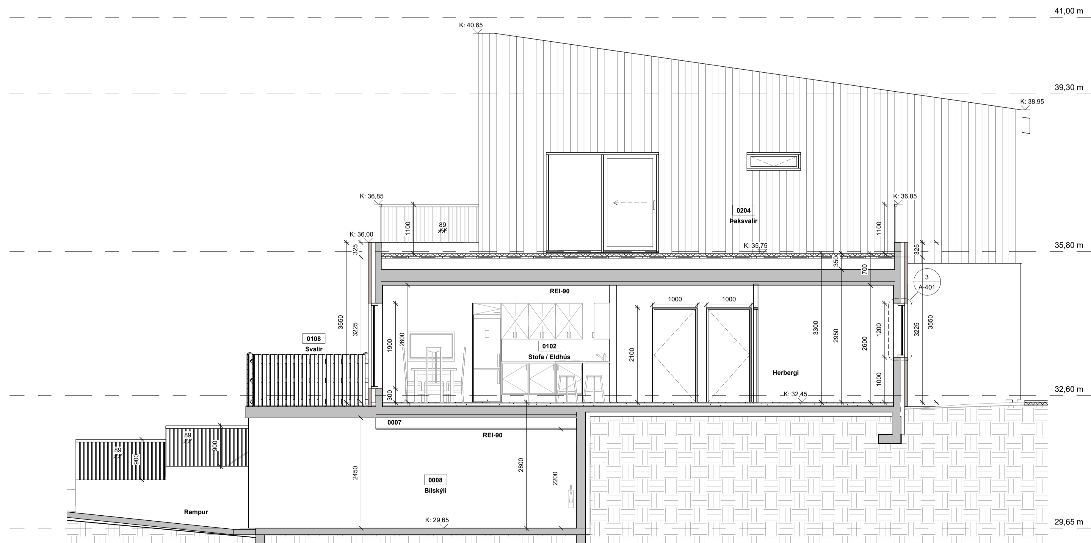
- SNID C 1 : 50
