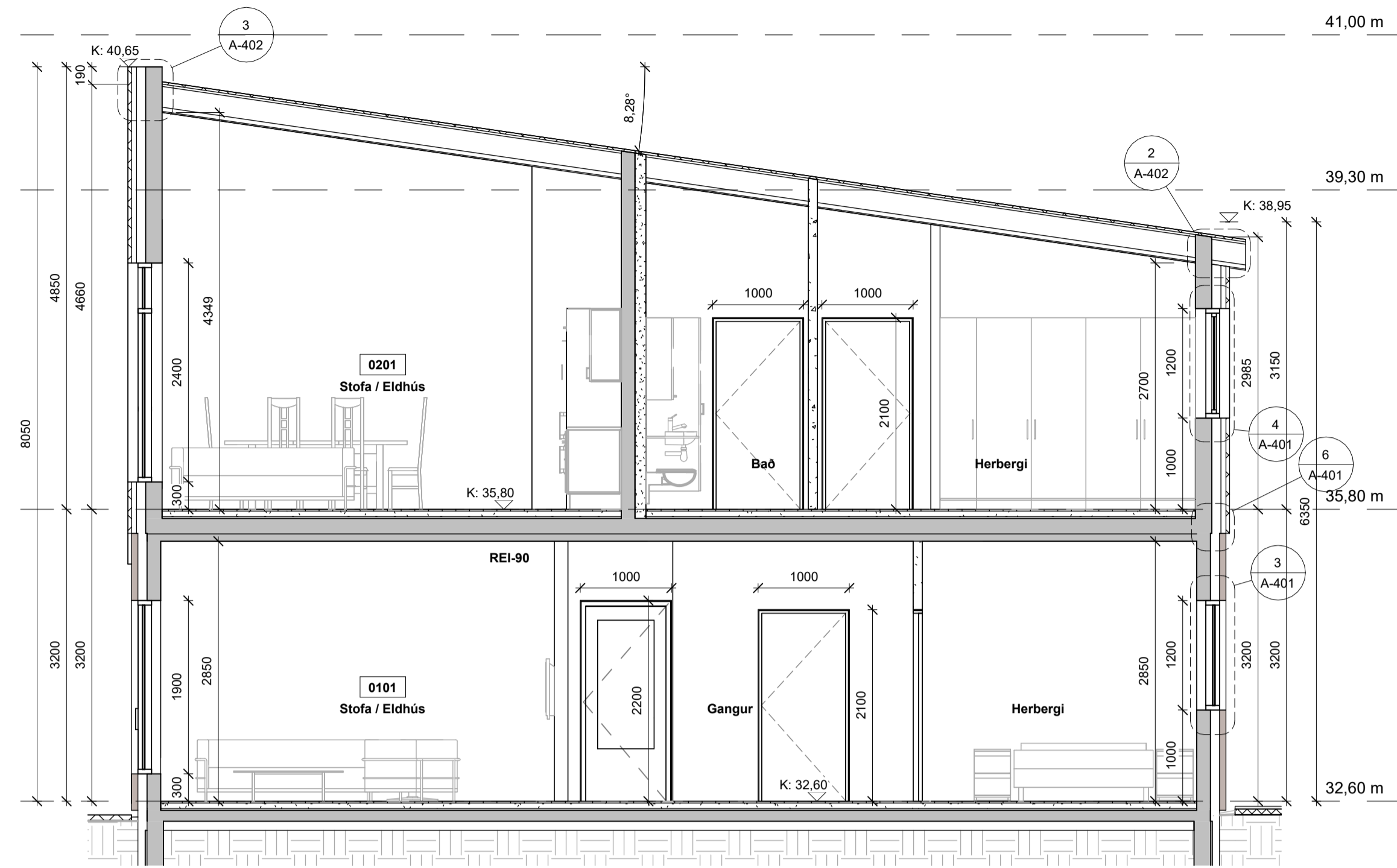
- SNID B 1 : 50
